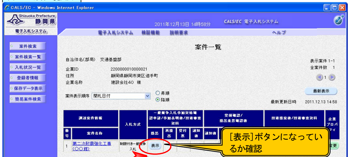
図9-16. 案件一覧画面
